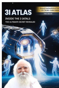
3i Atlas
